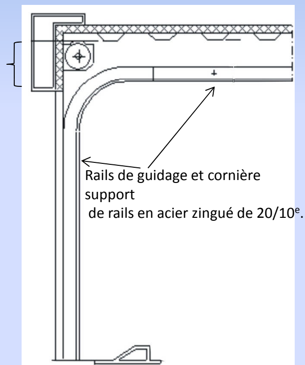
Equilibreur avec 2 ressorts galvanisé. Arbre en acier galvanisé !
